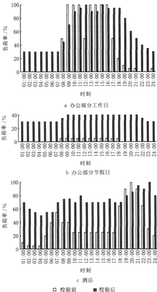
图 2 校验前后办公部分和酒店的照明和设备的负荷率
