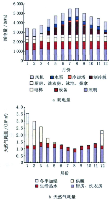
图 5 模型逐月耗电量与天然气耗量的分解
