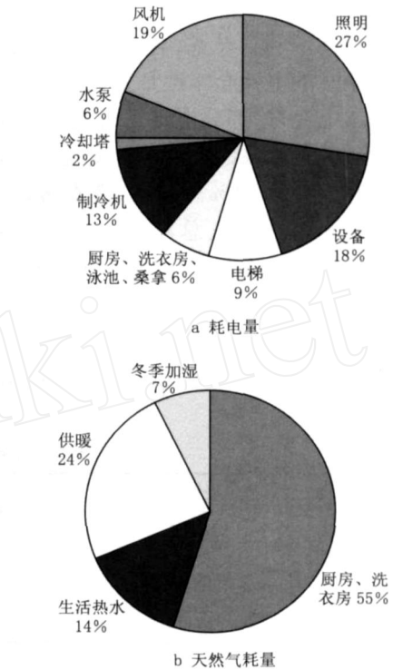
图 4 模型全年耗电量与天然气耗量的分解
