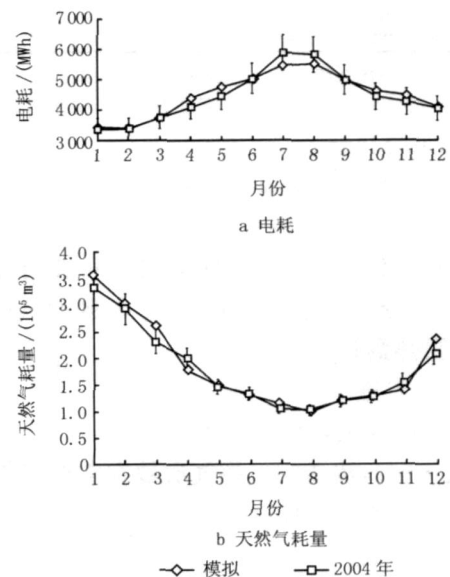
图 3 校验后的能耗模拟结果与 2004 年实际能耗的比较
