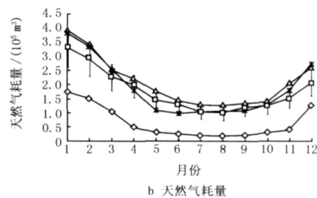
图 1 初次模拟的总能耗结果与 2002—2004 年实际能耗的比较
